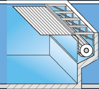
8. Abschirmplatte und Nischenabdeckungsbügel
